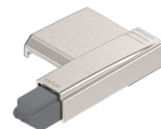
Závěs 170°
