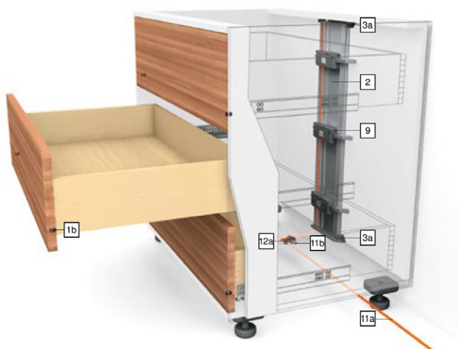
Korpus s vloženými čely
