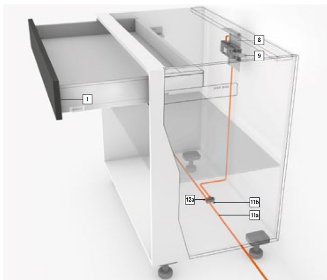
Korpus s jedním výsuvem - horní upínací úhelník
